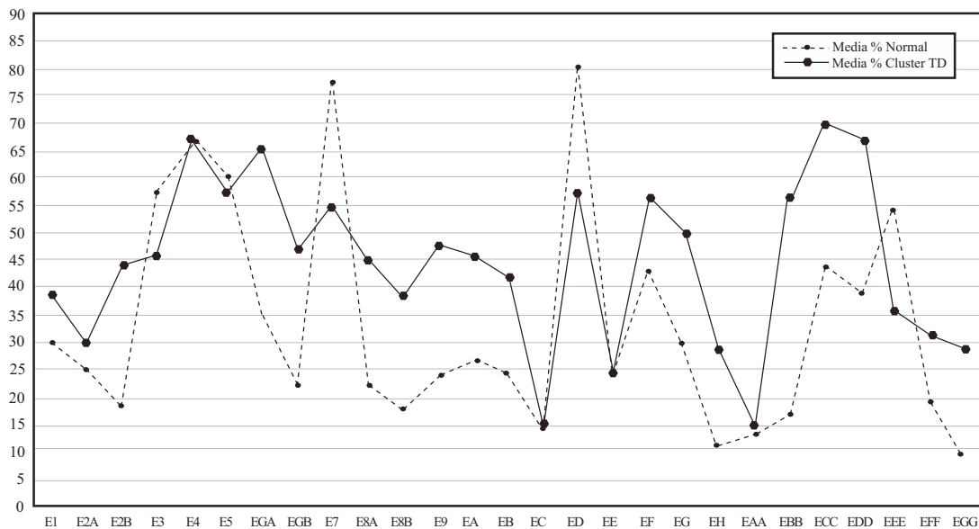
Figura 3. Gráfico del conglomerado Tipo I (T-D).
