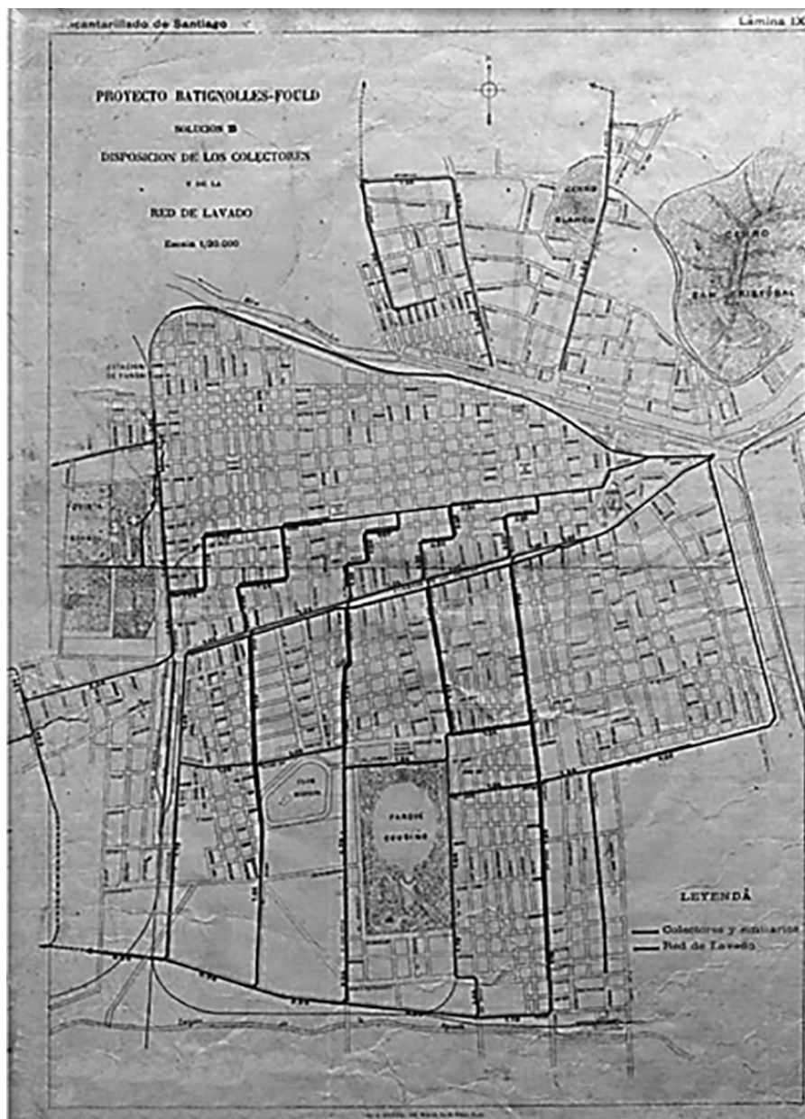
FIGURA 4 Plano de Santiago del Proyecto B de la Société de Construction des Batignolles et MM. Fould y Cie. (1904) [colectores y emisarios (gris claro), red de lavado (gris oscuro)]
